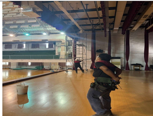
侷限型偵煙探測器訊號回路配置施工中
