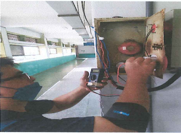
火警標示燈回路量測無異常
